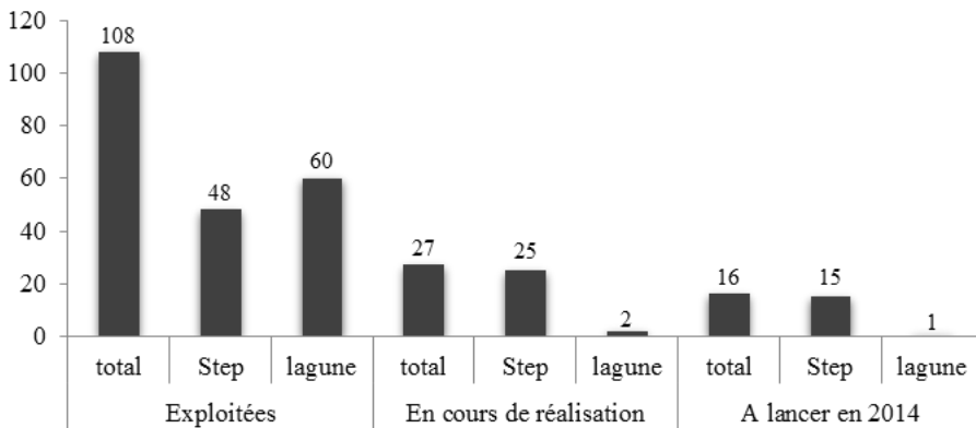
Figure 1 : Données des stations d'épuration en Algérie.
