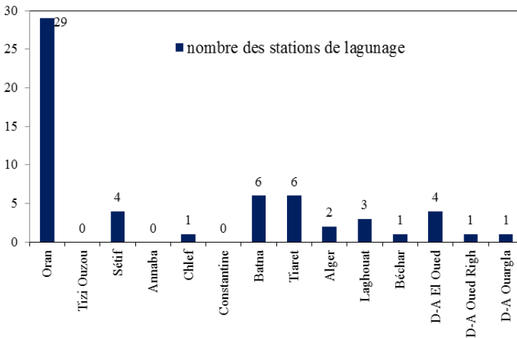
Figure 4 : Répartition géographique des stations de lagunage en Algérie (Source : établi à partir des données de ONA (1), 2014).
