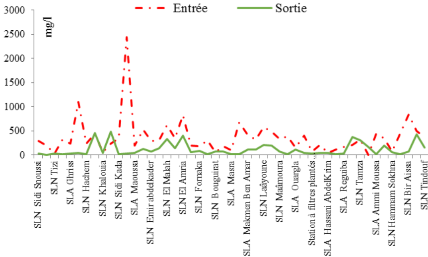
Figure 2 : Valeurs des MES dans les stations de lagunage en Algérie.
