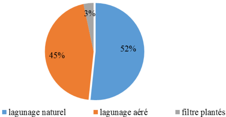
Figure 3 : Typologie des stations de lagunages en Algérie.
